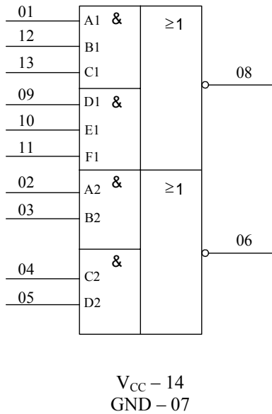
Условное графическое обозначение
